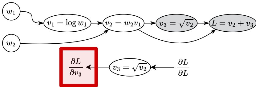
Рисунок 20. Иллюстрация обратного режима автоматического дифференцирования
