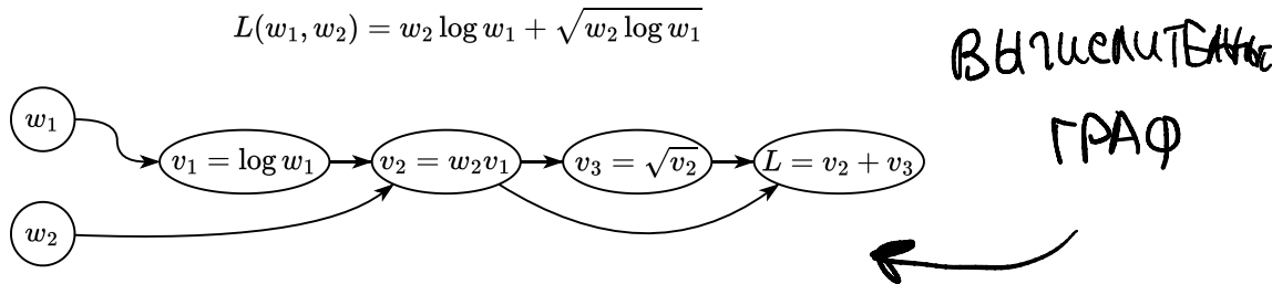
Рисунок 6. Иллюстрация вычислительного графа для функции L(w_1, w_2)
