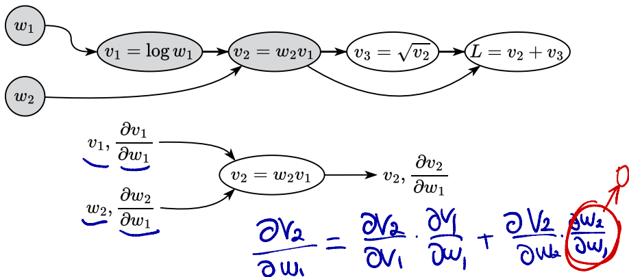
Рисунок 9. Иллюстрация прямого режима автоматического дифференцирования
