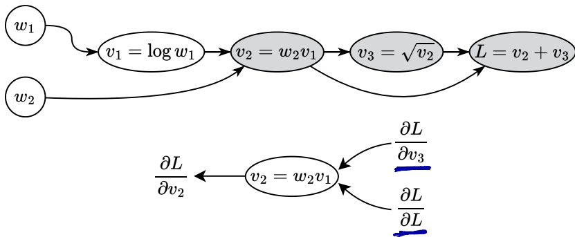
Рисунок 21. Иллюстрация обратного режима автоматического дифференцирования
