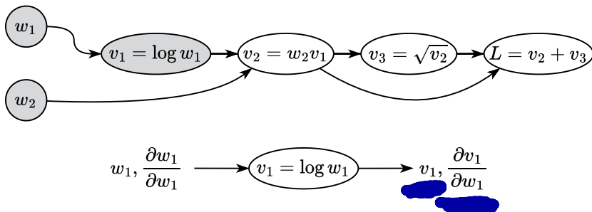
Рисунок 8. Иллюстрация прямого режима автоматического дифференцирования
