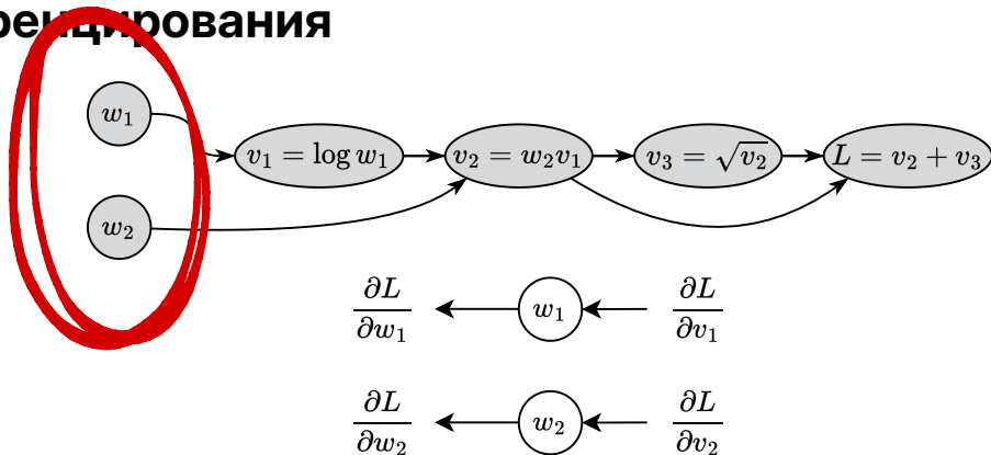
Рисунок 23. Иллюстрация обратного режима автоматического дифференцирования
