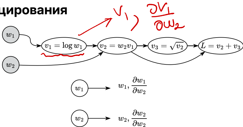
Рисунок 13. Иллюстрация прямого режима автоматического дифференцирования
