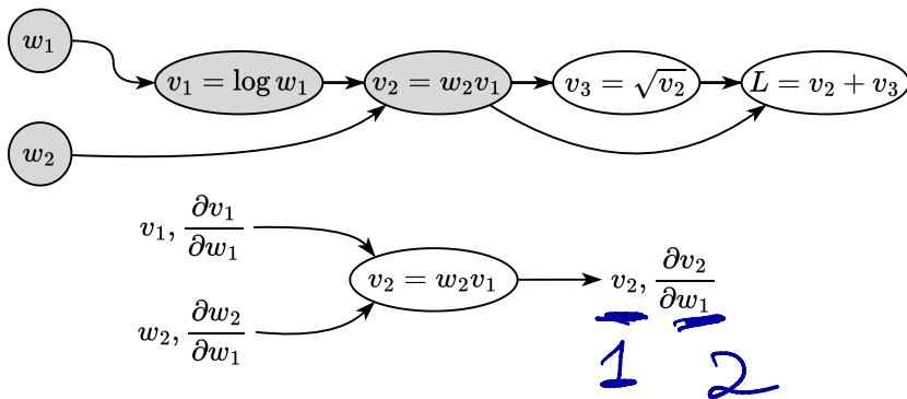
Рисунок 9. Иллюстрация прямого режима автоматического дифференцирования
