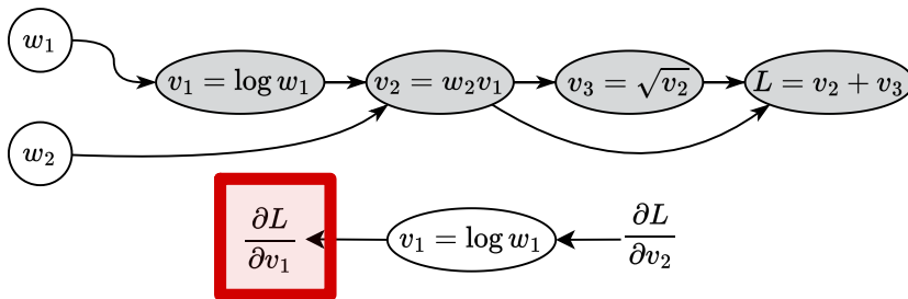
Рисунок 22. Иллюстрация обратного режима автоматического дифференцирования
