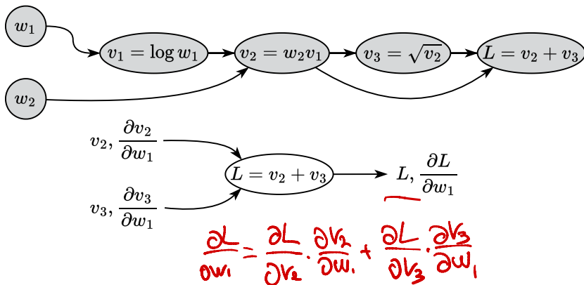
Рисунок 11. Иллюстрация прямого режима автоматического дифференцирования
